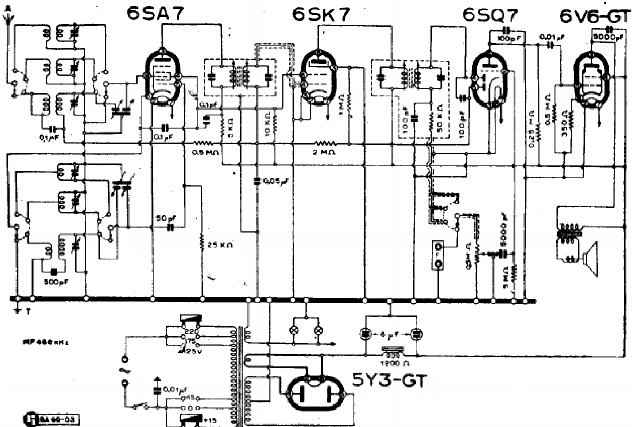
MELI RADIO - MOD. « MR 2620-S »
